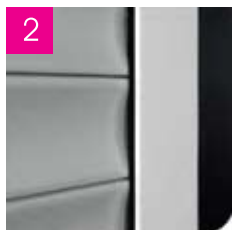
Coulisses 95 x 34 mm équipées de joints brosse intérieurs et extérieurs avec film d'étanchéité.
